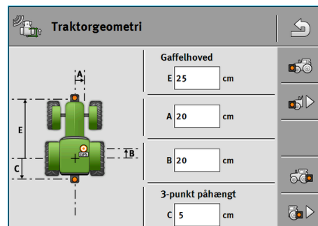
Eksemplarisk traktorgeometri
