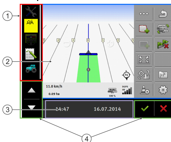
Områder på skærmen
