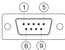
9-polet SUB-D-stik
