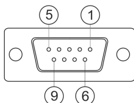
9-polet SUB-D-bøsning
