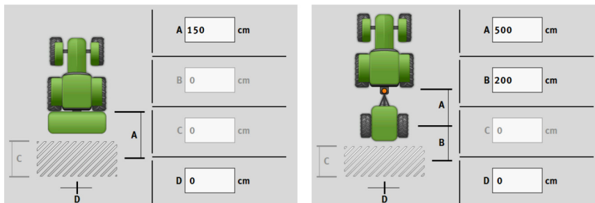
Maske til indtastning af geometrien ved forskellige maskinmodeller
