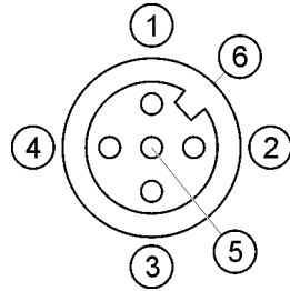
M12-bøsning: Ethernet
